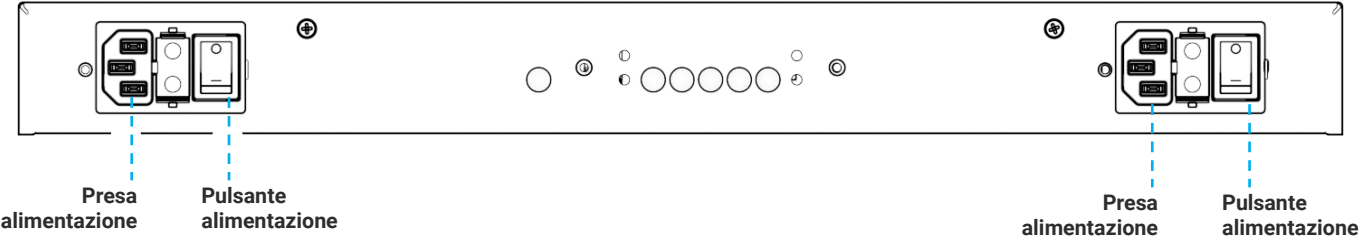
Vista retro
