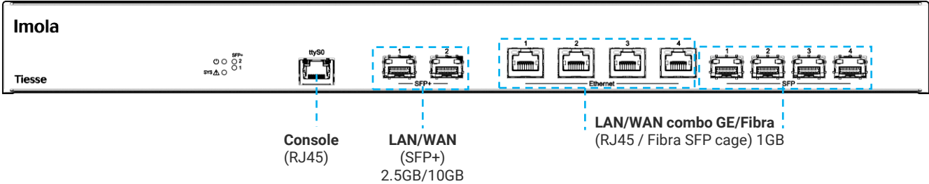
Vista retro
